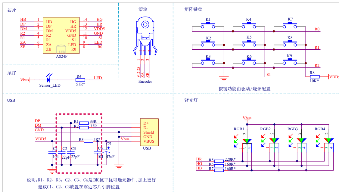
图 3. 应用电路图
