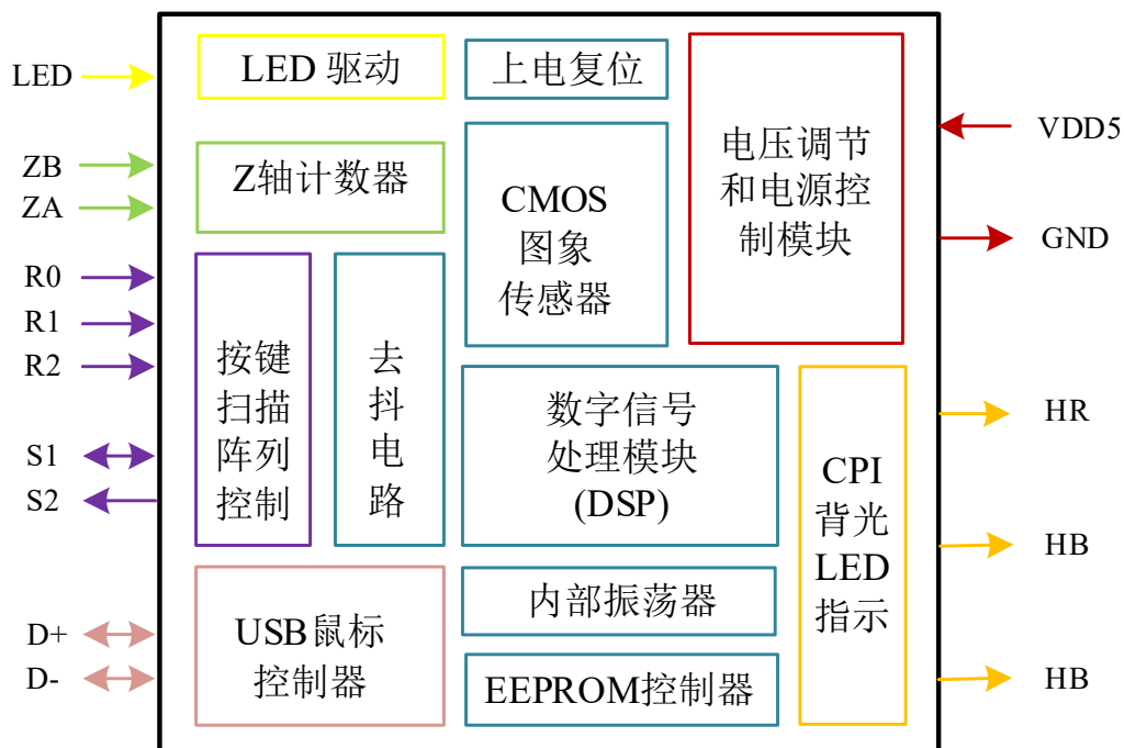
图 2. 模块框图
